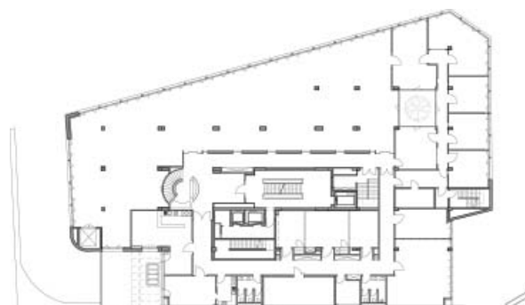
Plan du rez supérieur
