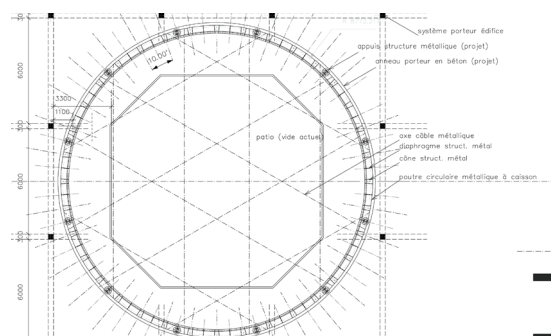
Plan et coupe de principe - Blue office architecture
