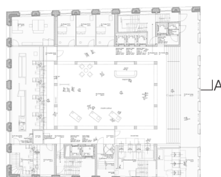
Plan du rez-de-chaussée
