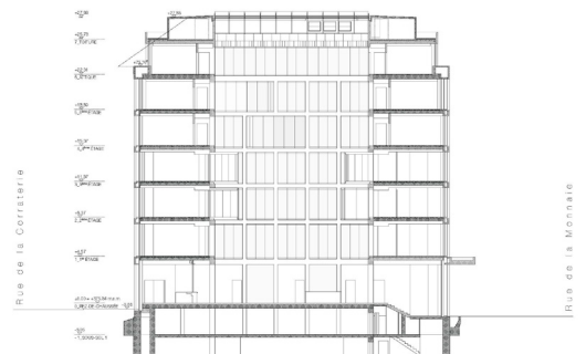
Coupe A-A
