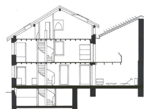
Coupe longitudinale
